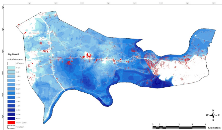
รูปที่ 2.15 ระดับความสูงน้ำท่วมและอาคารในเขตผังเมืองรวมพุนพินปี 2554 (ที่มา: วารัตน์ และคณะ, 2556)
