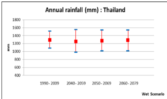
รูปที่ 3.7 การเปลี่ยนแปลงปริมาณฝนรายปีเฉลี่ยและปริมาณฝนสูงสุด-ต่ำสุดในรอบ 20 ปี ในอนาคตเมื่อเทียบกับช่วงปีปัจจุบัน (ค.ศ.1990-2009)
