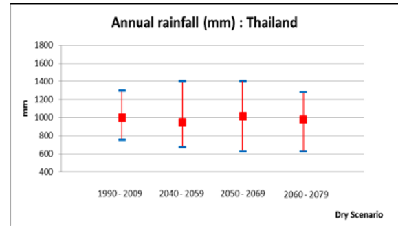
รูปที่ 3.7 การเปลี่ยนแปลงปริมาณฝนรายปีเฉลี่ยและปริมาณฝนสูงสุด-ต่ำสุดในรอบ 20 ปี ในอนาคตเมื่อเทียบกับช่วงปีปัจจุบัน (ค.ศ.1990-2009)
