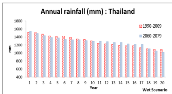
รูปที่ 3.6 การเปลี่ยนแปลงปริมาณฝนรายปีเมื่อเทียบปีที่มีฝนมากที่สุดไปถึงปีที่มีฝนน้อยที่สุดในรอบ 20 ปี (ค.ศ.2060-2079) เมื่อเทียบกับช่วงปีปัจจุบัน (ค.ศ.1990-2009)
